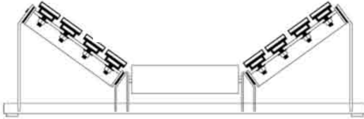
Typowy widok wzdłużny rynny trójkrażnikowej
